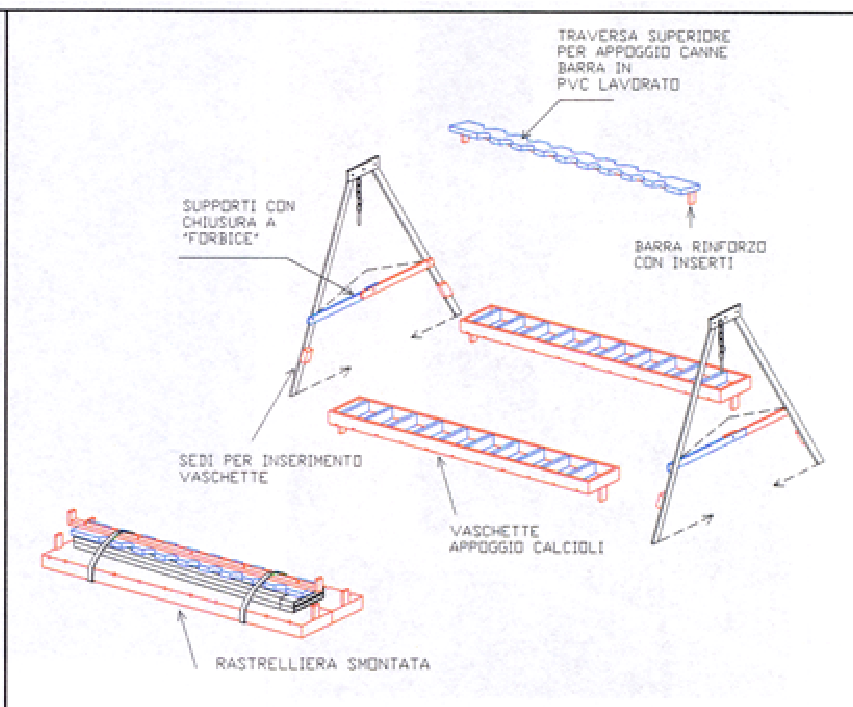
Rastrelliere scomposta ed imballata
