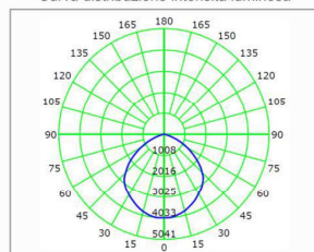
Curva distribuzione intensità luminosa
