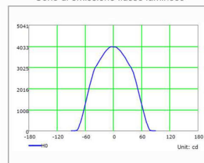
Cono di emissione flusso luminoso
