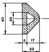
sez. 40x22
