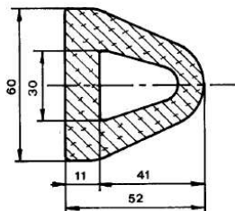
sez. 60x52
