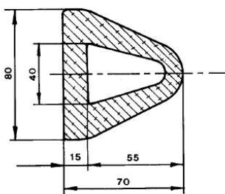
sez. 80x70
