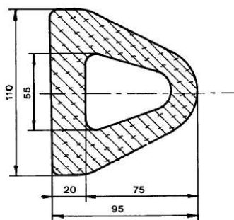
sez. 110x95
