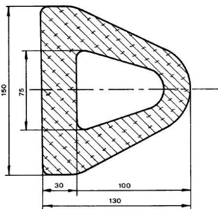
sez. 150x130
