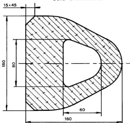
sez. 150x160
